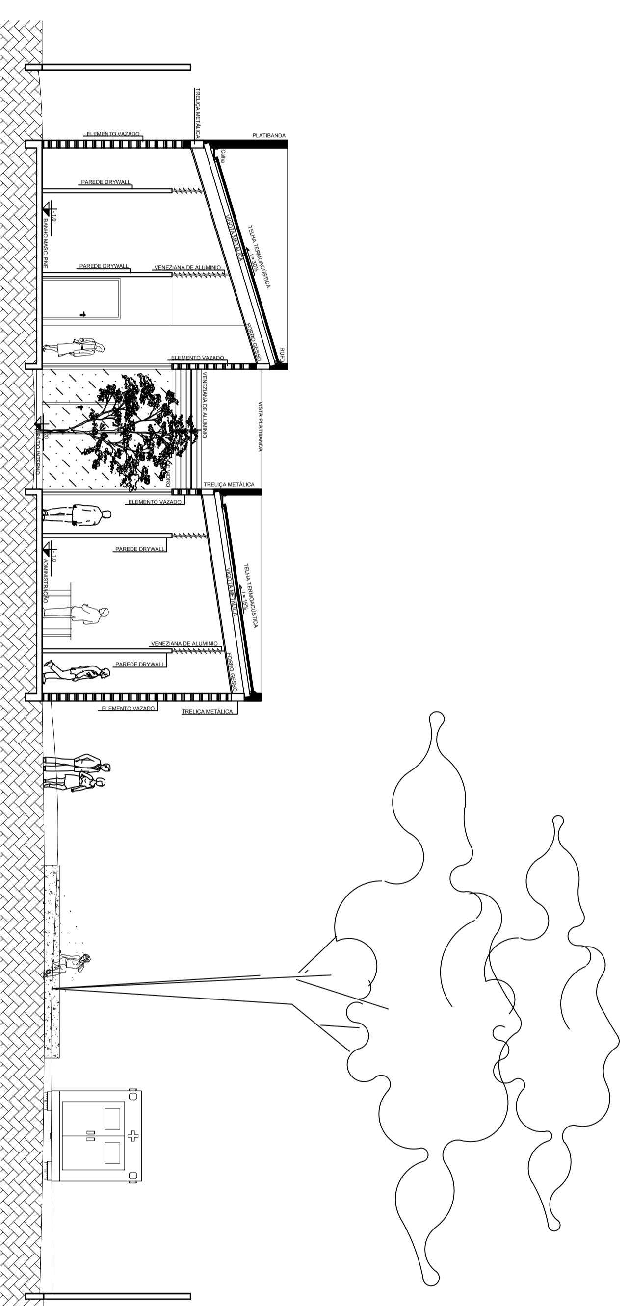
04 CORTE AA esc: 1/100
